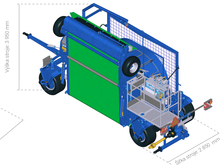
Rozměry v přepravní poloze
