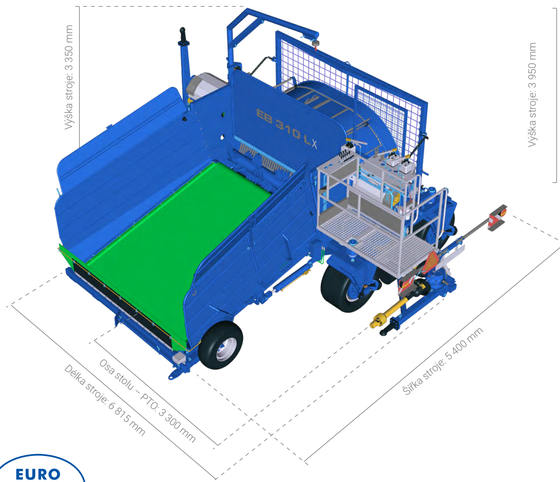
Rozměry v pracovní poloze
